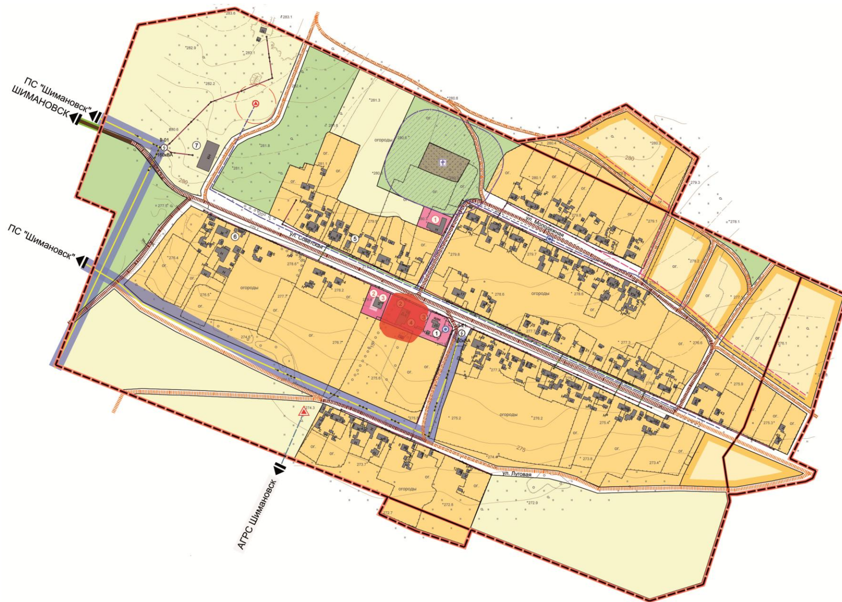
Рис. 2.1 – Зона действия котельной "ДК".
